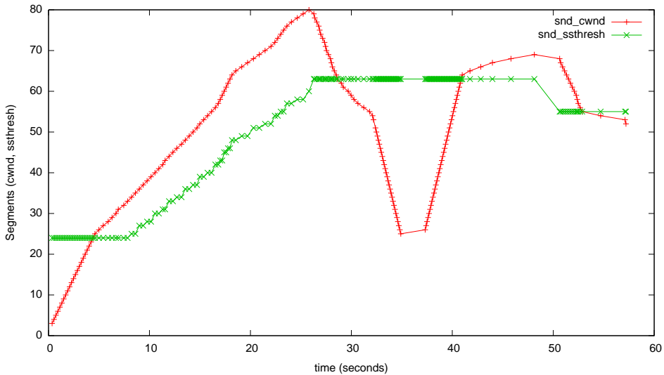
myTcpProbeData - bic-mode=1
