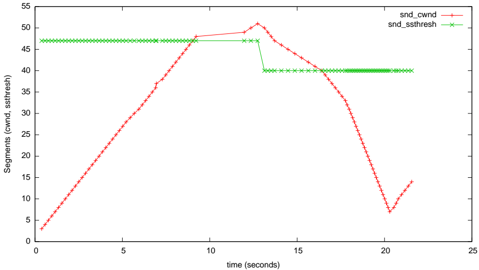
myTcpProbeData - bic-mode=2b
