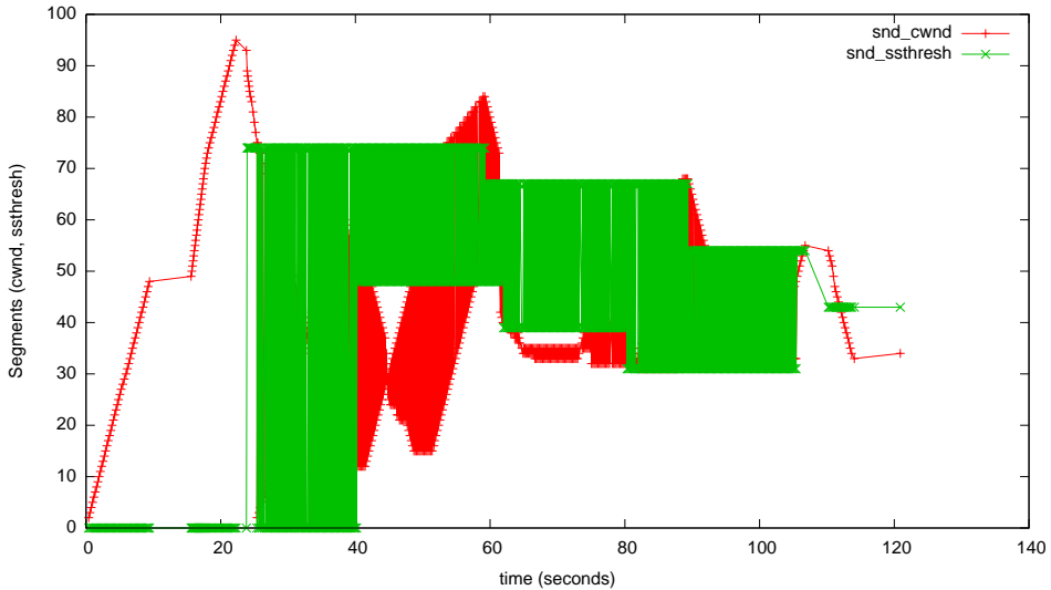
myTcpProbeData - bic-mode=3
