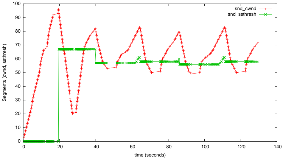
myTcpProbeData - cubic-mode=1
