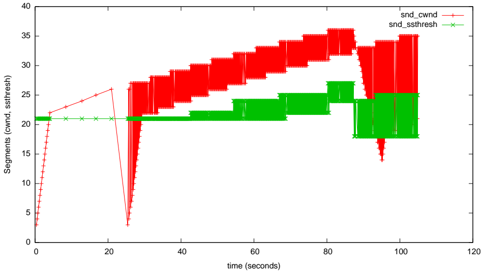
myTcpProbeData - highspeed-mode=3
