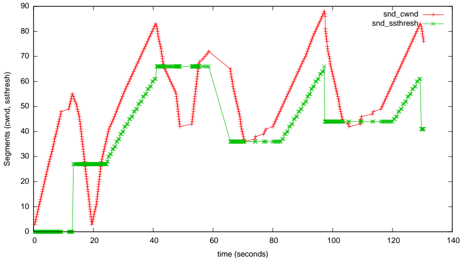
myTcpProbeData - htcp-mode=2b
