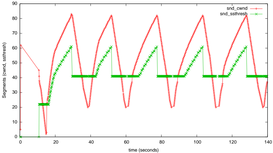
myTcpProbeData - hybla-mode=1
