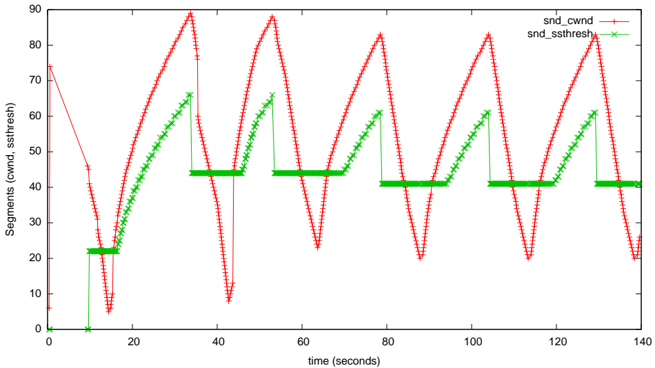
myTcpProbeData - hybla-mode=2
