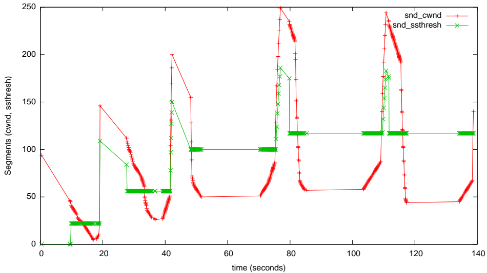
myTcpProbeData - hybla-mode=2b
