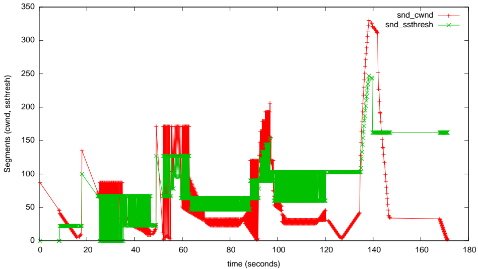
myTcpProbeData - hybla-mode=3
