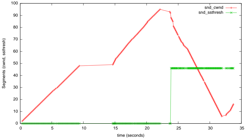
myTcpProbeData - illinois-mode=2
