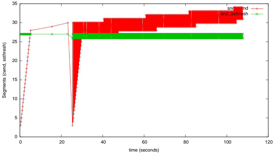
myTcpProbeData - illinois-mode=3
