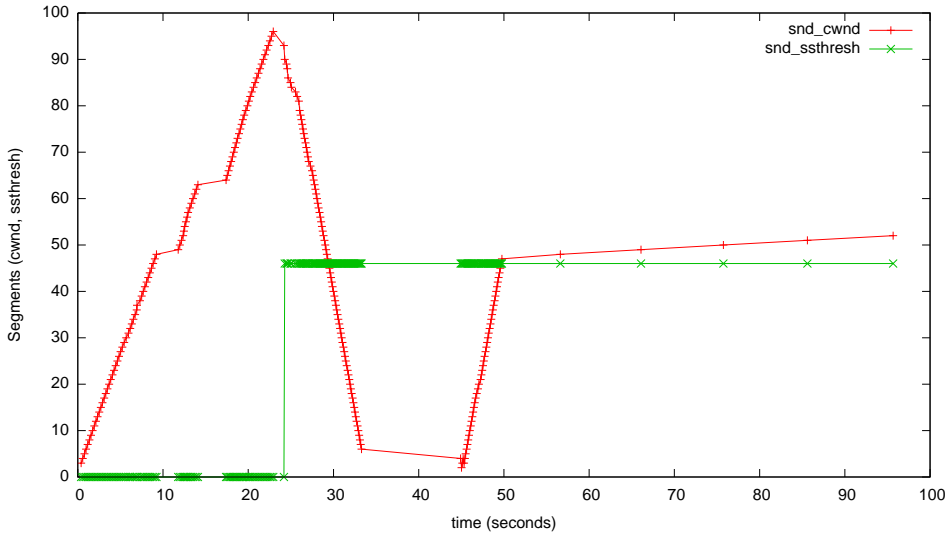
myTcpProbeData - reno-mode=2
