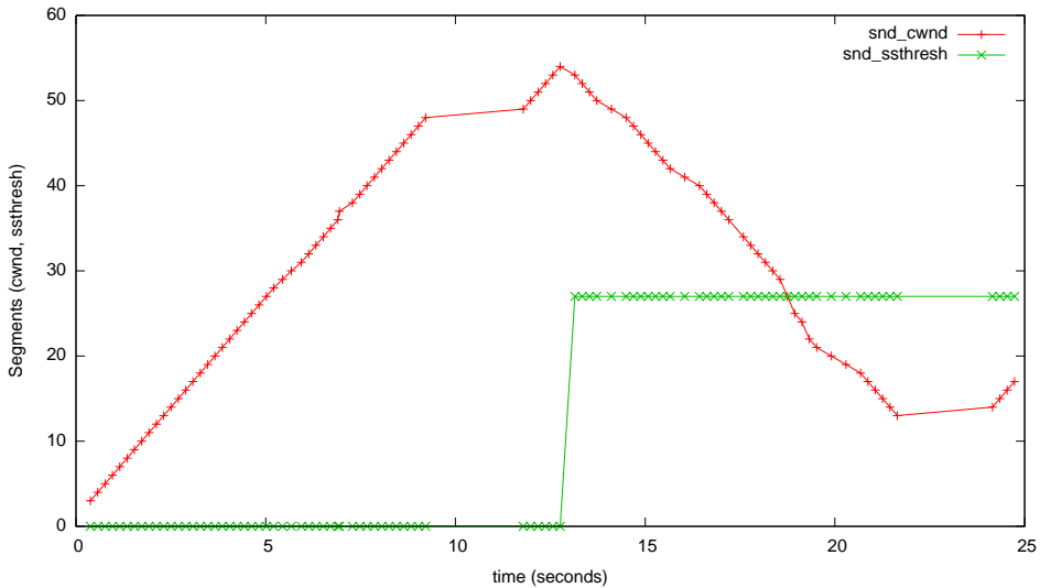
myTcpProbeData - reno-mode=2b
