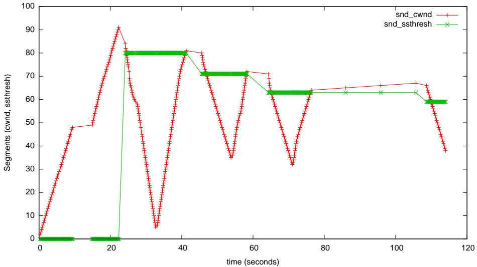
myTcpProbeData - scalable-mode=2
