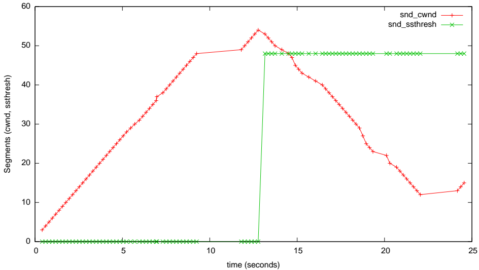
myTcpProbeData - scalable-mode=2b
