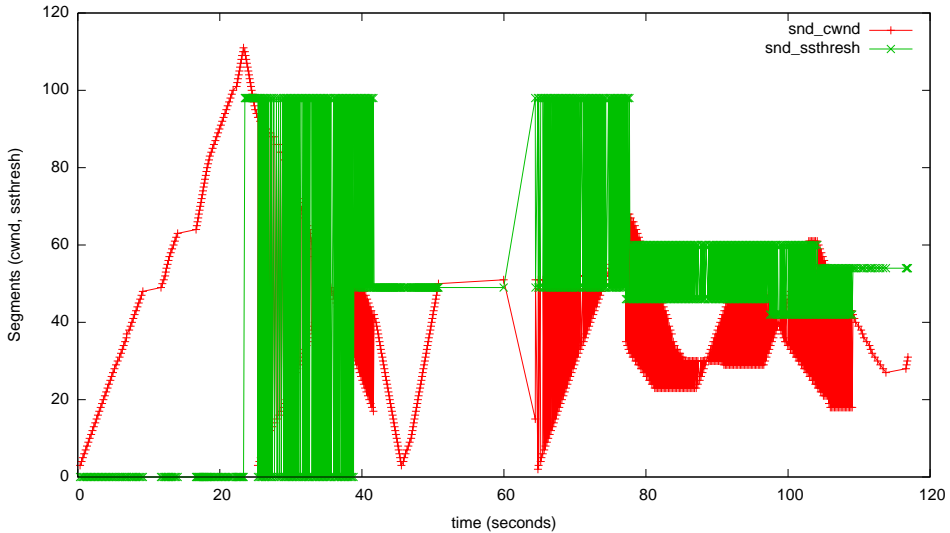
myTcpProbeData - scalable-mode=3
