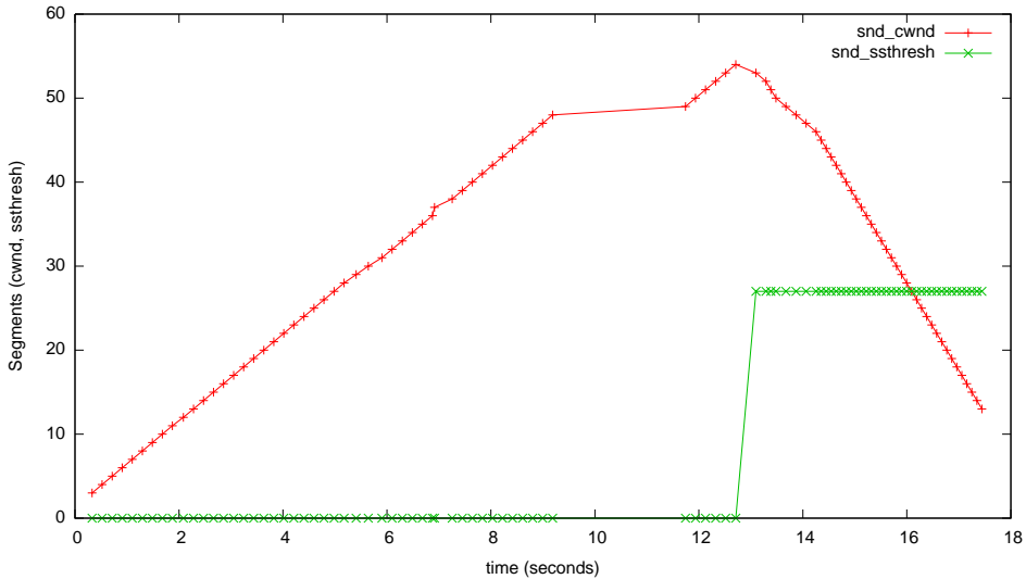
myTcpProbeData - veno-mode=2b
